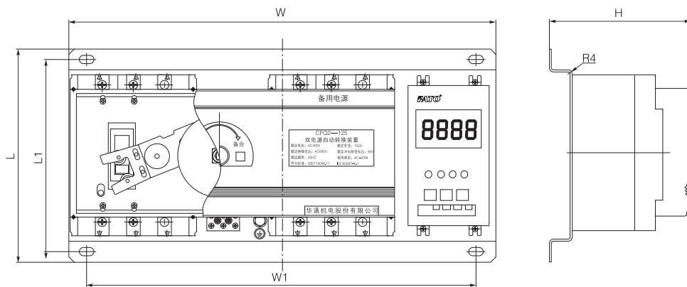
图7 CFQ2一体式
