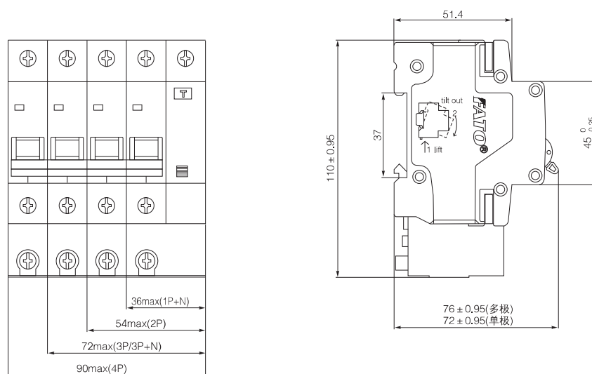
图1 CFB1NLE-63外形及安装尺寸
